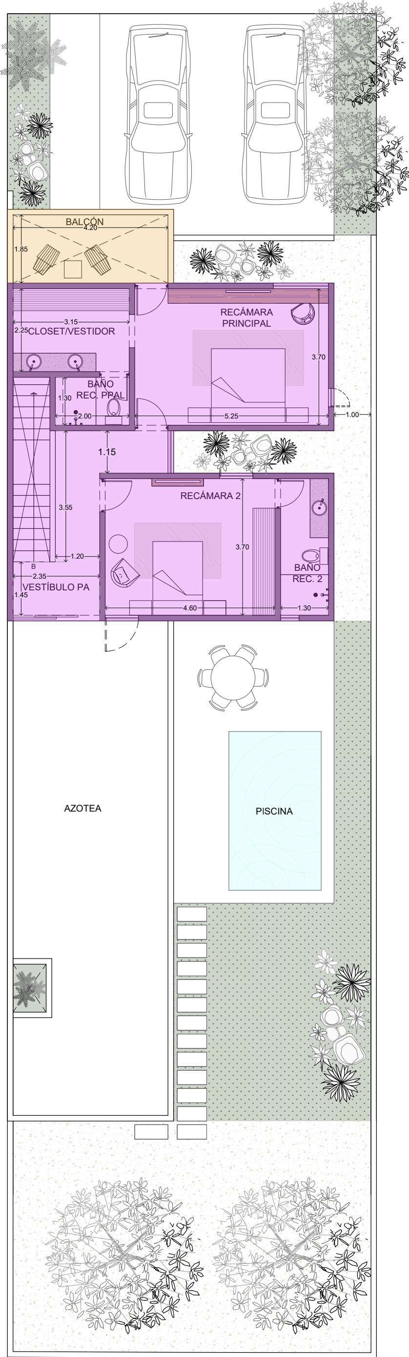
PLANTA ALTA
