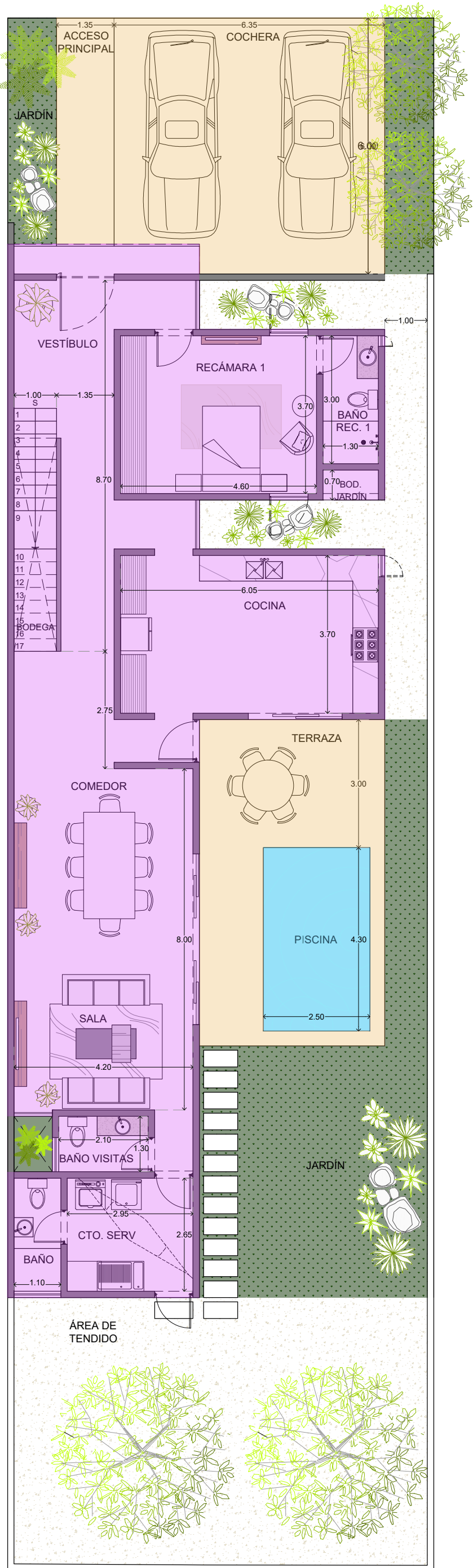
PLANTA BAJA
