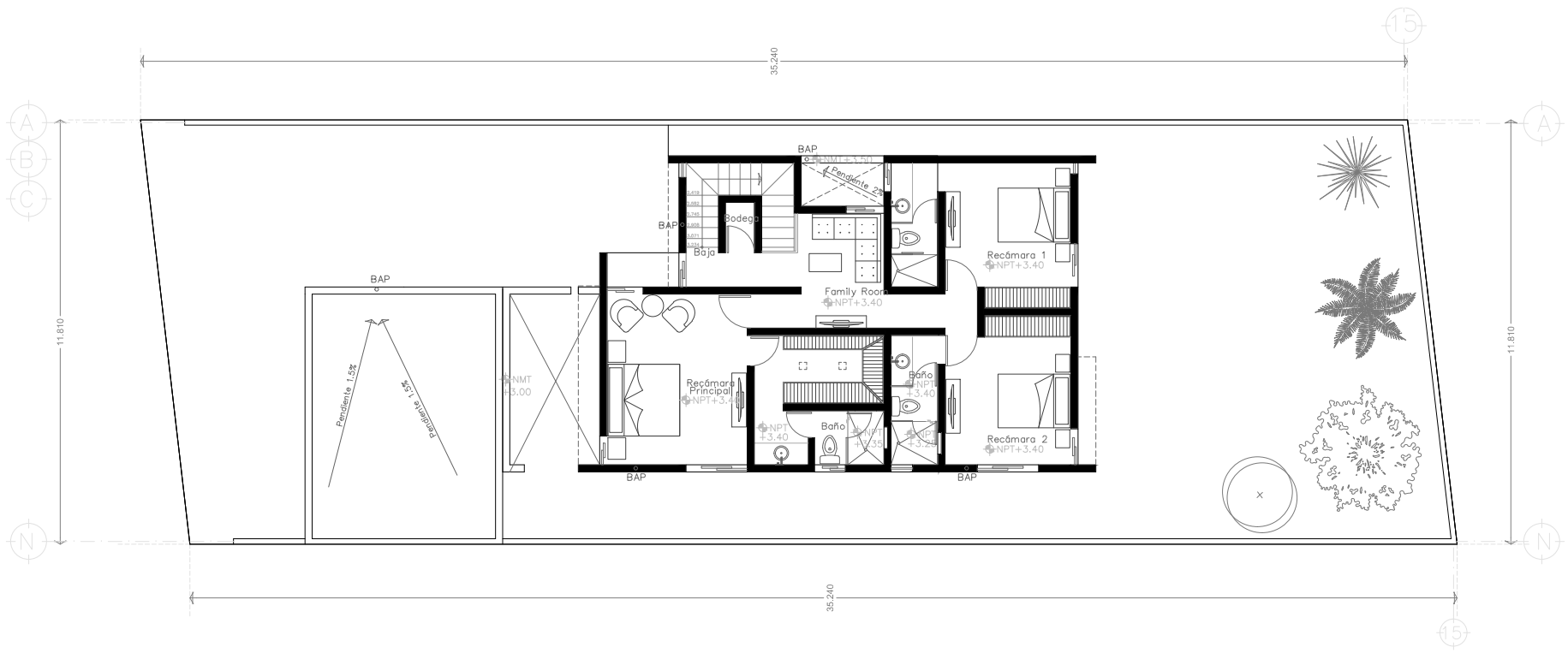
PLANTA ALTA
