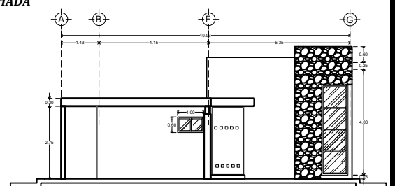
FACHADA
