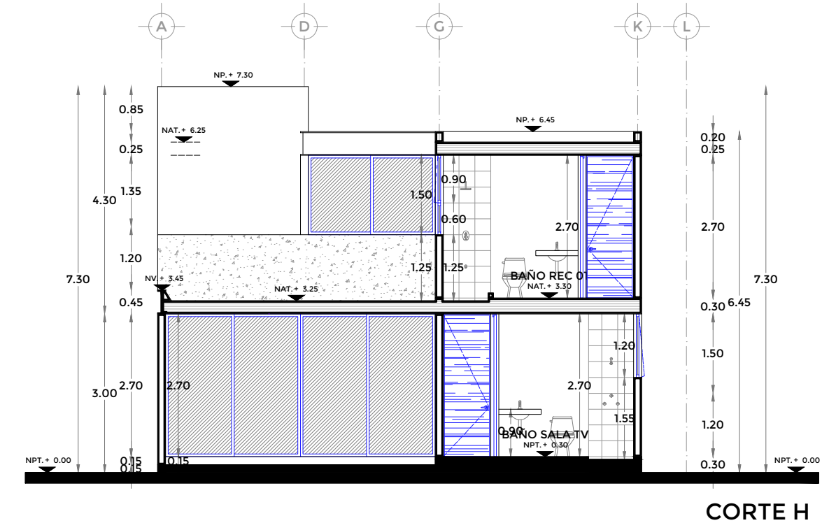
CORTE H
