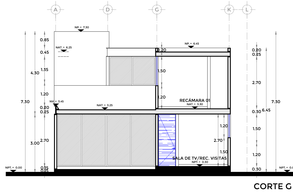
CORTE G
