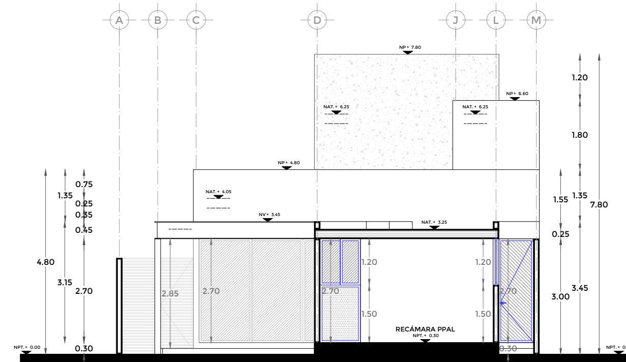
CORTE G
