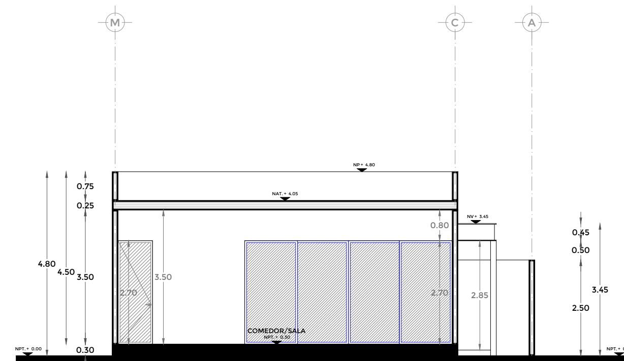
CORTE K
