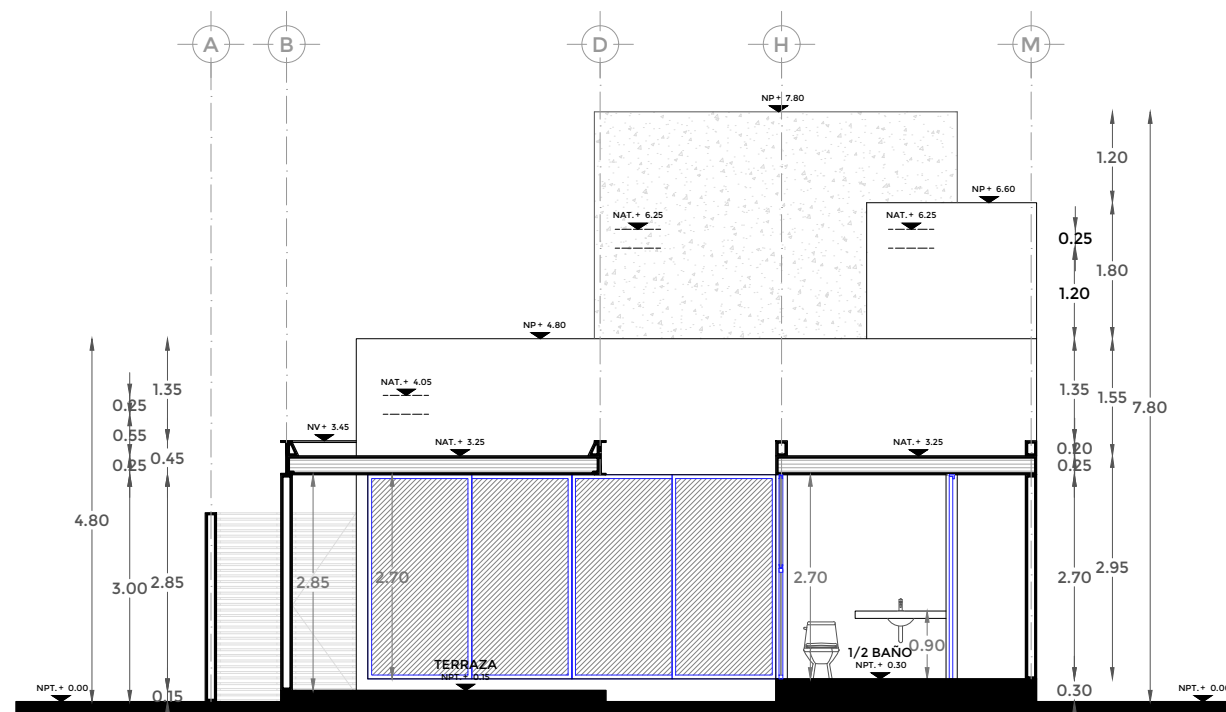
CORTE J
