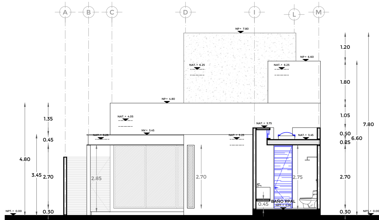
CORTE F
