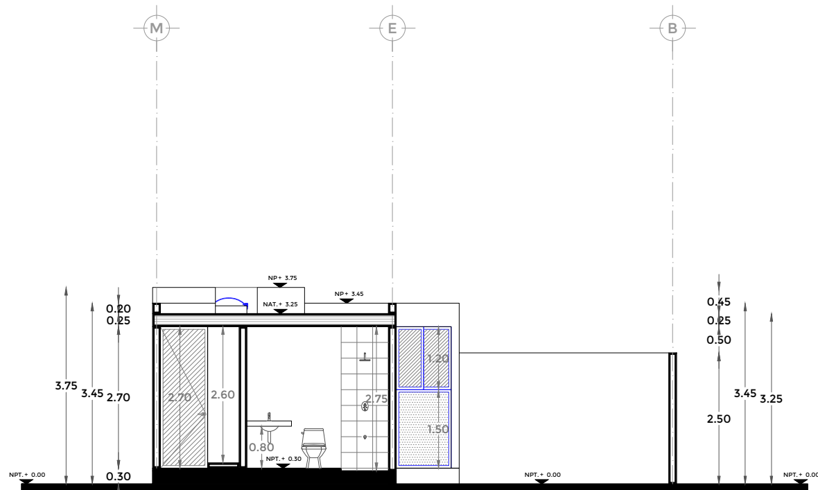
CORTE H
