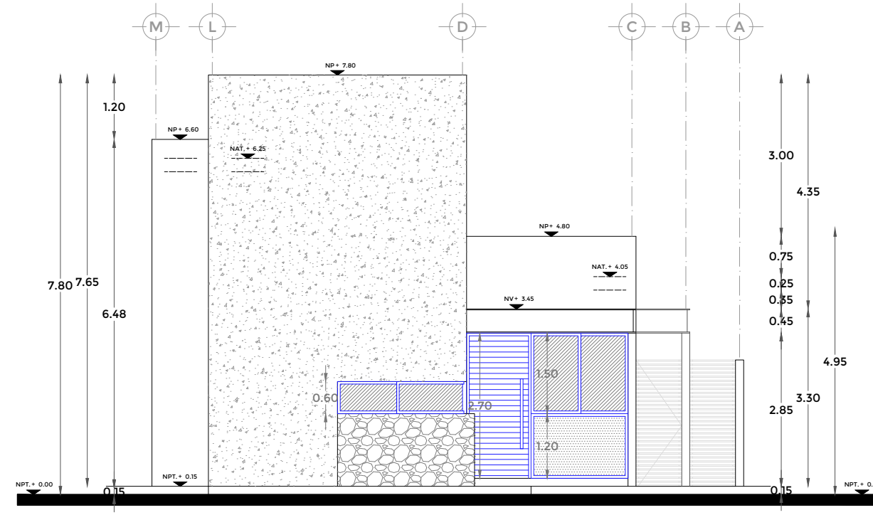
FACHADA
