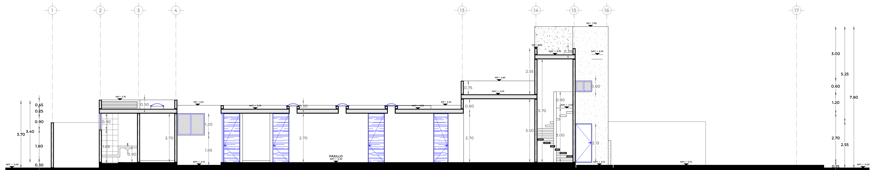
CORTE A
