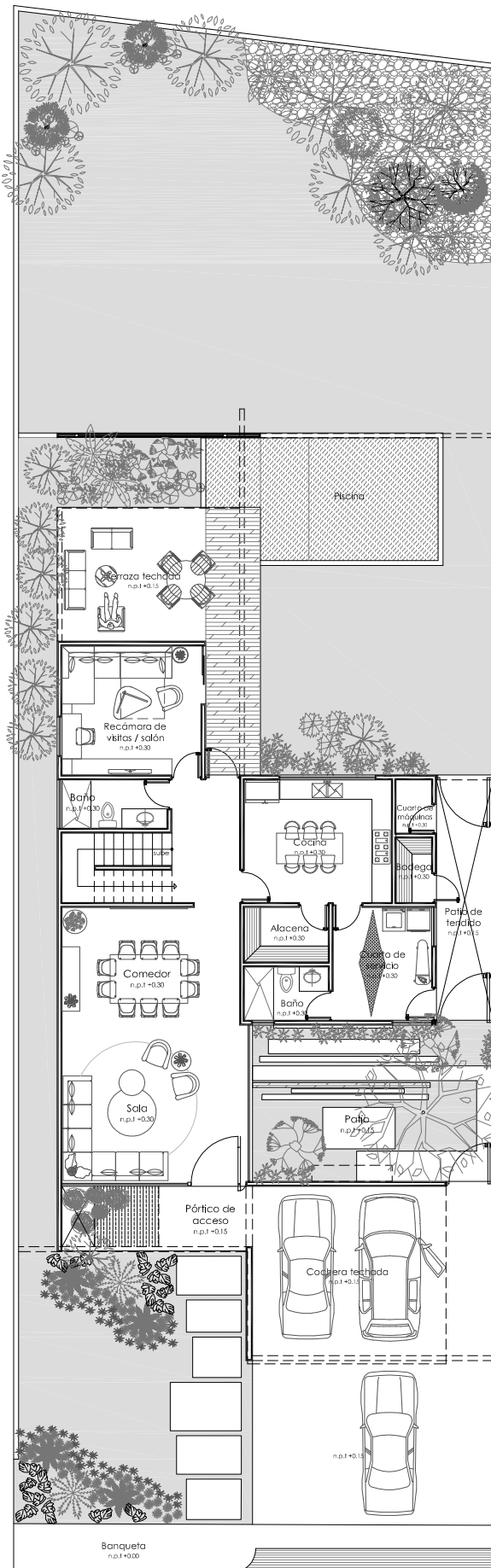
Planta arquitectónica baja
