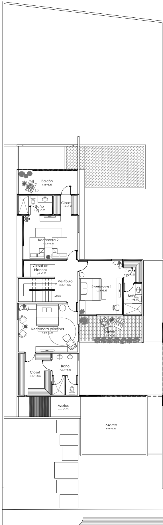
Planta arquitectónica alta
