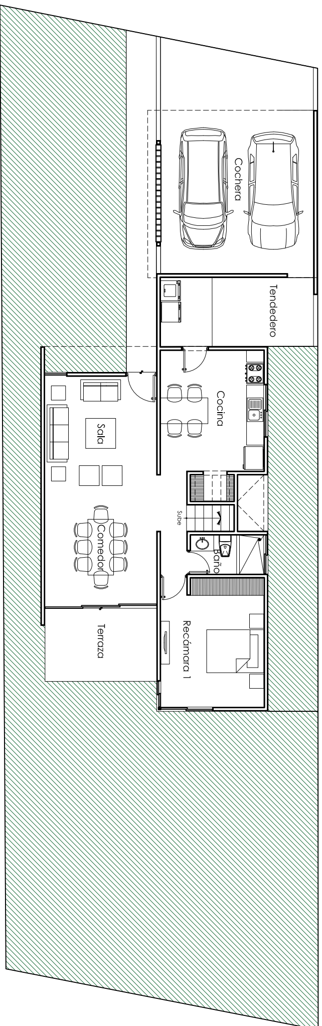
PLANTA BAJA
