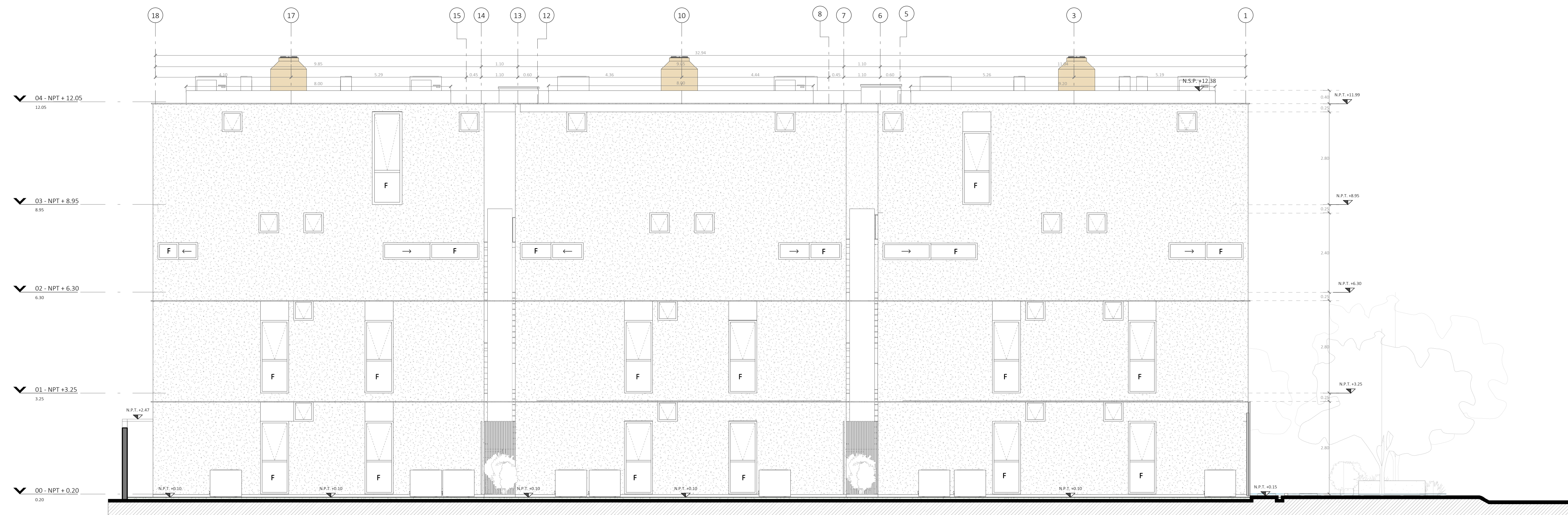
FACHADA ESTE ESC 1 : 75
