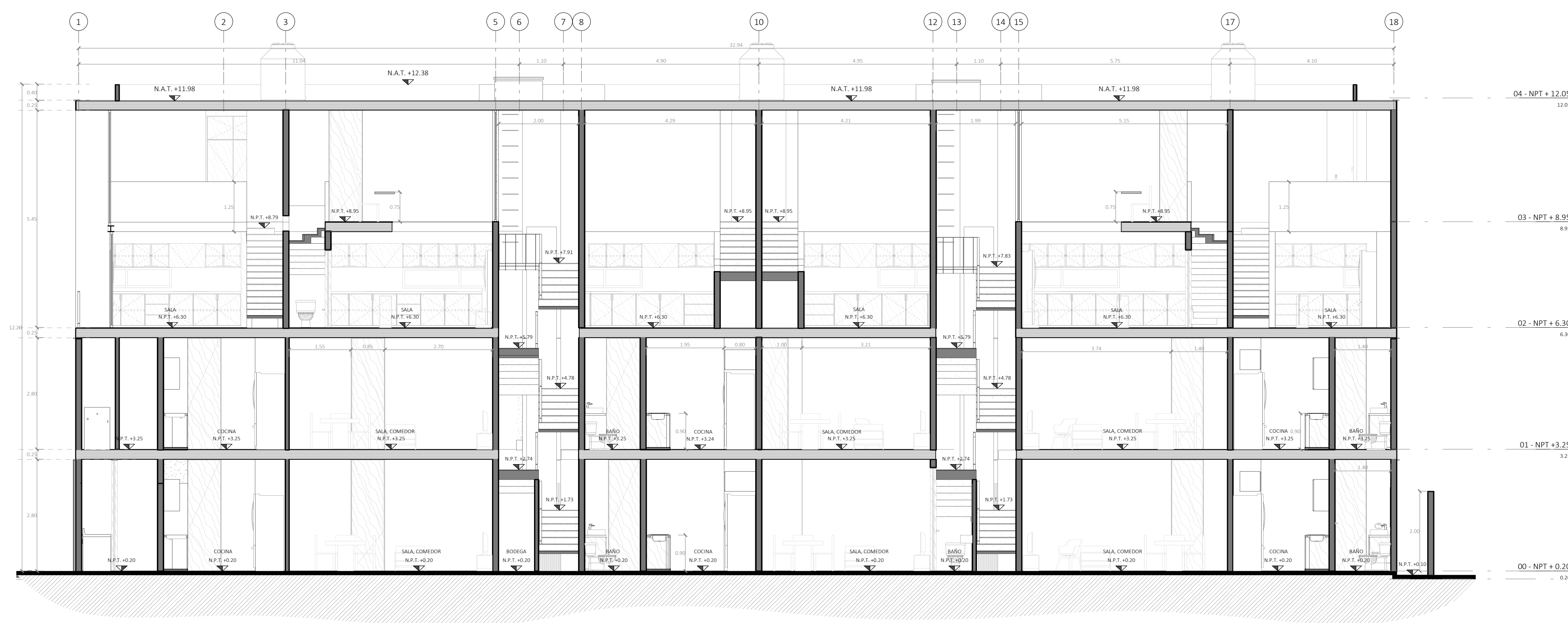
2 | CORTE ARQUITECTÓNICO 2 ESC 1 : 75
